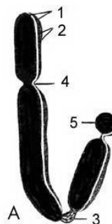
Схема строения митотической хромосомы, подпишите все ее составляющие
